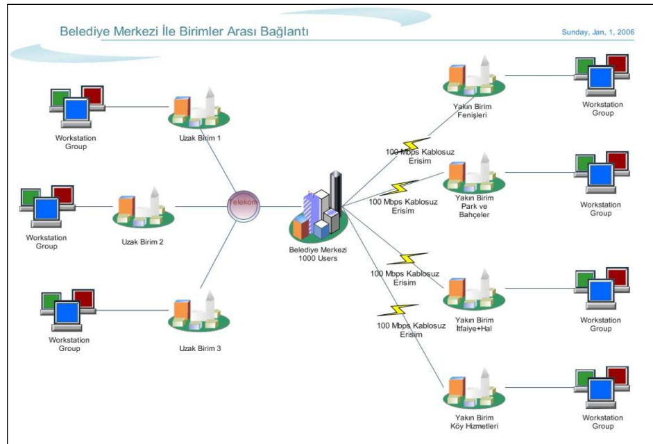
Belediye ve Dış Birimlerin Bağlantı Şeması
