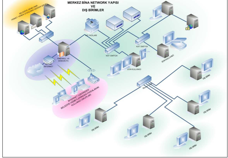
Belediye ve Dış Birimlerin Bağlantı Şeması
